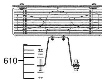
600 Additional Fan/Ventilation Additionelle/Zusatzfilter 75 Z EBM 601/602/603
